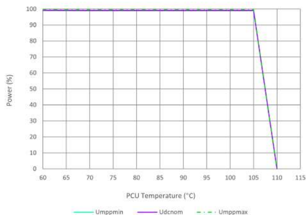
Puissance de déclasserement du micro-onduleur série MI VS. Température de la PCU
